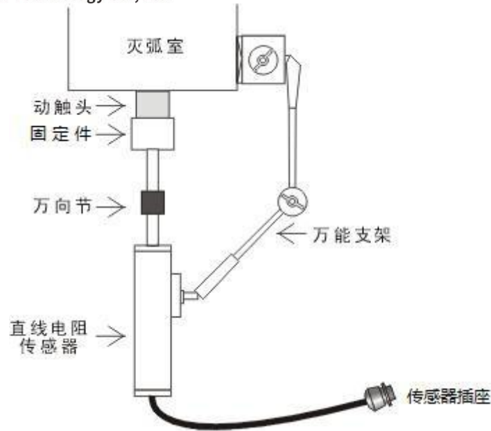
图14 行程传感器安装示意图
