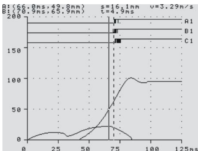
图6 时间-行程数据曲线图 操作提示：
