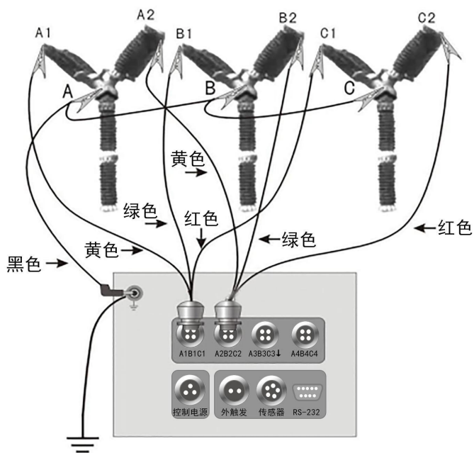
图10 六断口接线图
