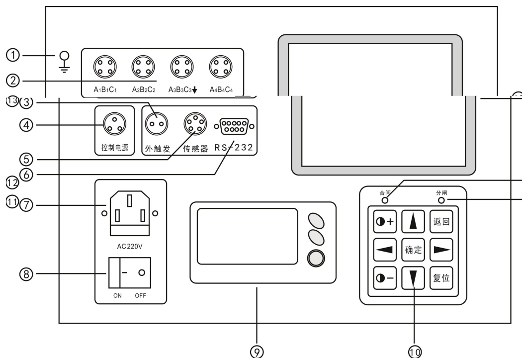
图1 面板布局图
